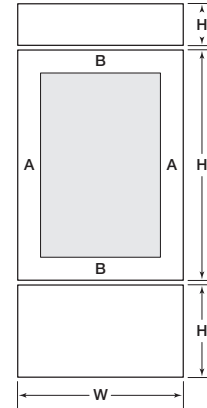
BI-30UG, BI-36UG
